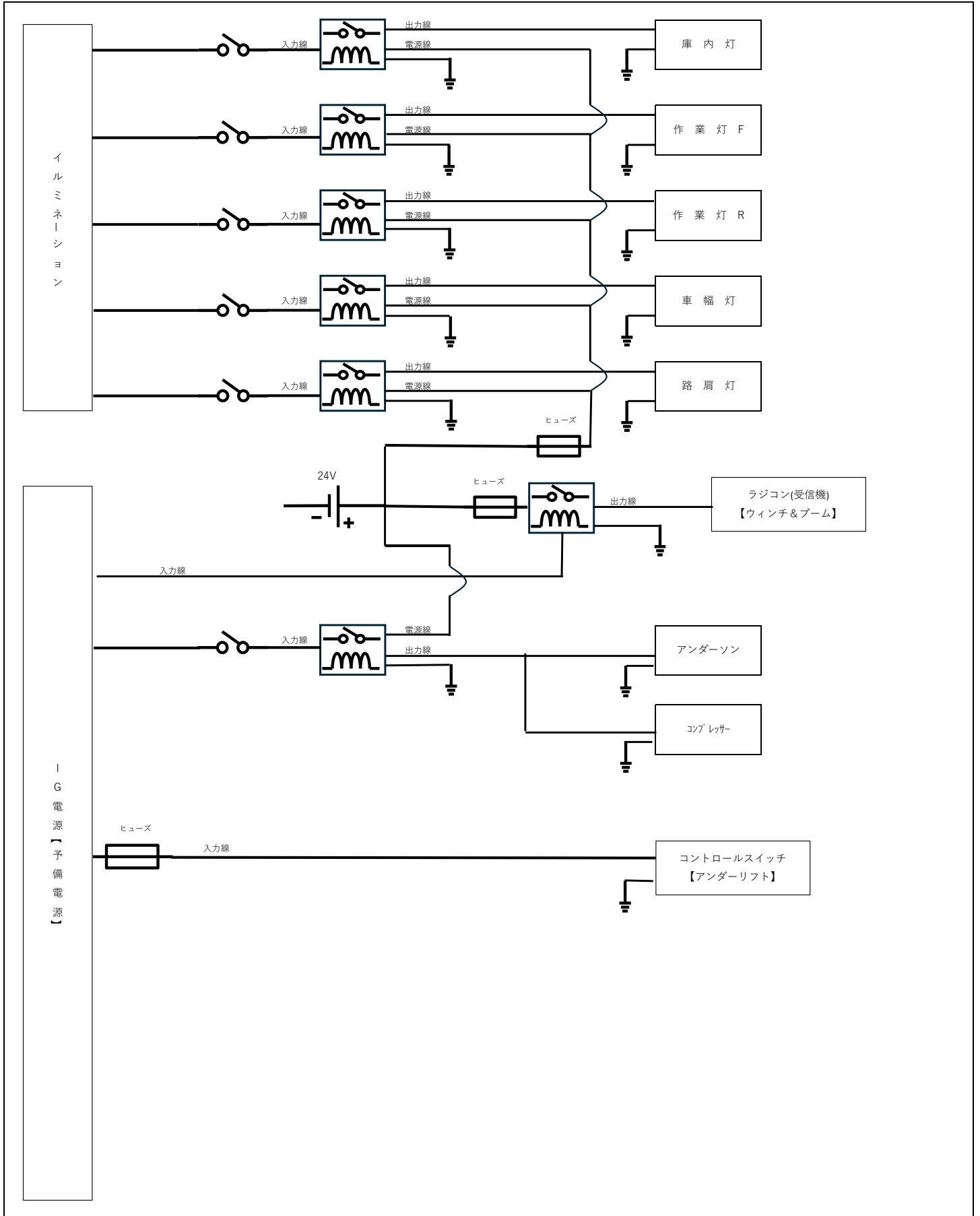
配線図
